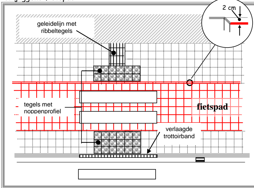
Aanliggend fietspad
